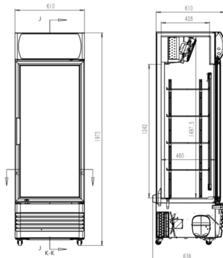
Sección Comercial
